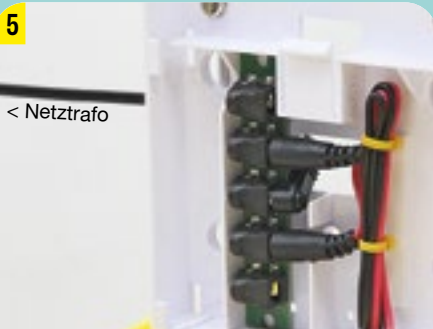
NETZKABEL VON HINTEN DURCH DIE ÖFFNUNG STECKEN UND MIT NIEDERVOLT-VERTEILER VERBINDEN (STECKPLATZ 3)
