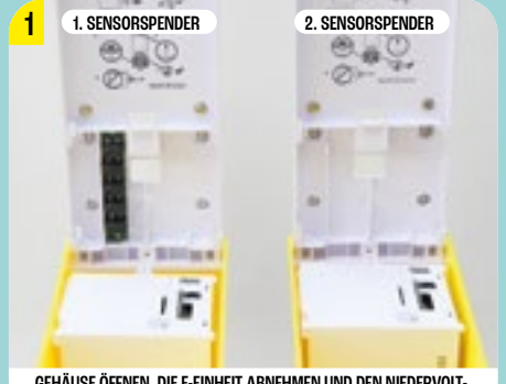
GEHÄUSE ÖFFNEN, DIE E-EINHEIT ABNEHMEN UND DEN NIEDERVOLT-VERTEILER IN DAS GEHÄUSE VON SENSORSPENDER 1 SETZEN
