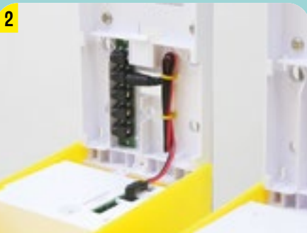
1. VERBINDUNGSKABEL MIT NIEDERVOLT-VERTEILER VERBINDEN (STECKPLATZ 2)
