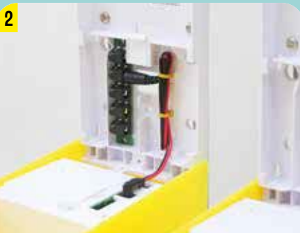
1. VERBINDUNGSKABEL MIT NIEDERVOLT-VERTEILER VERBINDEN (STECKPLATZ 2)
